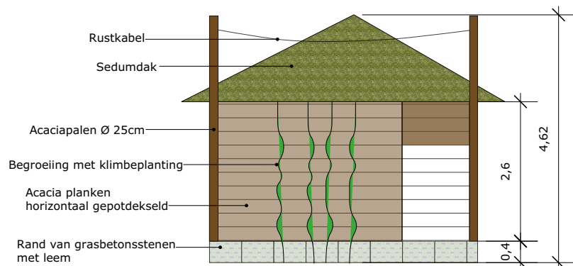
Vooraanzicht zuidzijde
