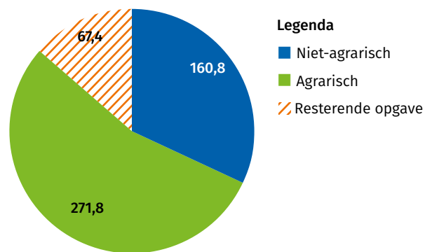
Figuur 19 Oppervlakte zonneparken in vergunningstraject, naar type grondgebruik (hectare) (bron: provincie Flevoland)
