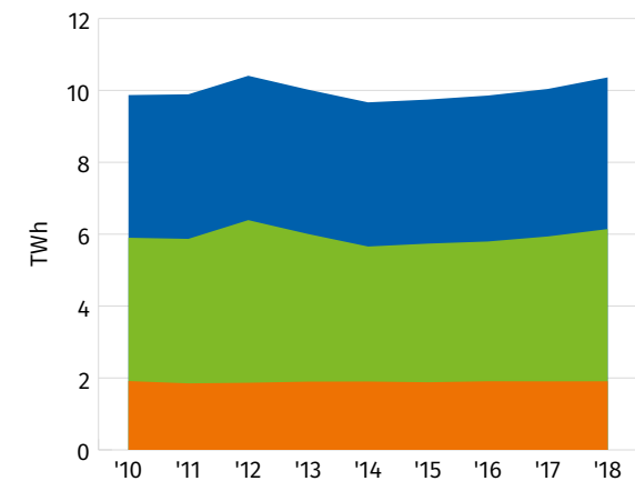
Figuur 5 Energiegebruik in Flevoland naar (secundaire) energiedrager (bron: Klimaatmonitor)
